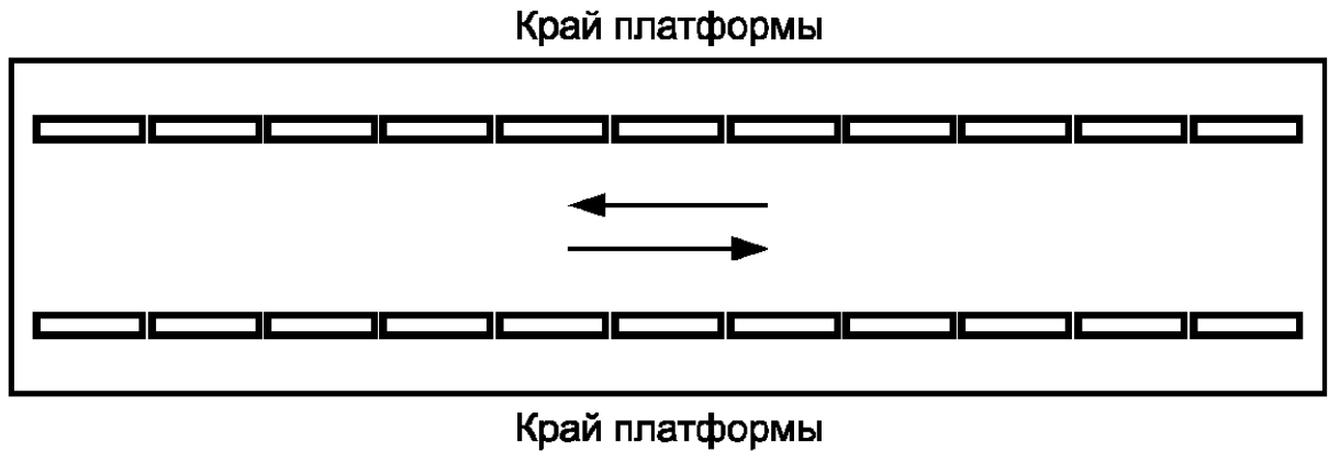
Рисунок А.4 - Форма рифления - одноэлементная тактильная полоса с плоской вершиной (шпунция), используемая для обустройства протяженных предупреждающих ТНУ вдоль края платформ различного назначения
